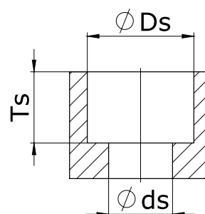
Зенкованное отверстие
