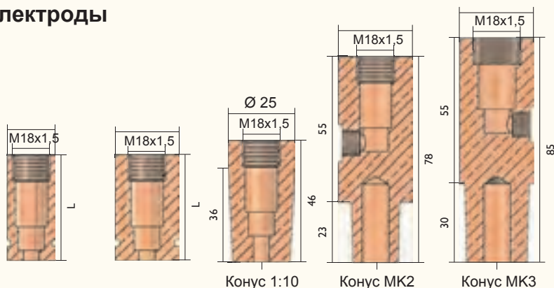
Конус 1:10 Конус МК2 Конус МК3
