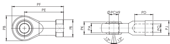
Чертёж / Technical Drawing
