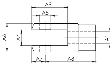
Чертёж / Technical Drawing
