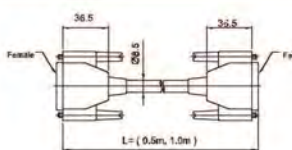
Двойной разъем MCS25-DC-5/10
