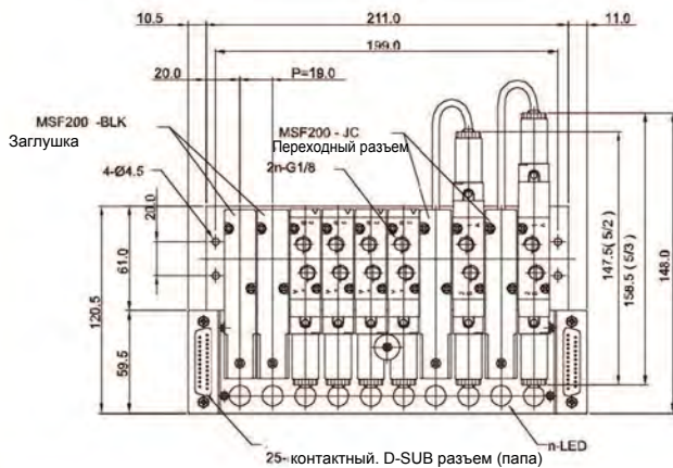
Двойной разъем MCS25-DC-5/10
