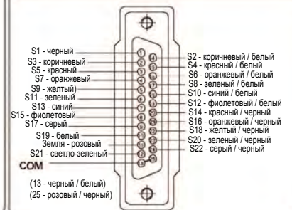
Заглушка MSF200 - BLK
