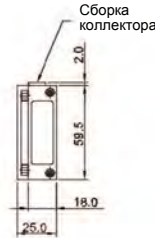
Одиночный модуль MCS211-T10-D4
